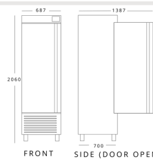
INFRICO AN501TF H 2060mm W 687mm D 700mm
