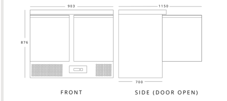
BLIZZARD BCC2 H 876mm W 903mm D 700mm
