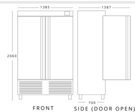
INFRICO AN1002TF H 2060mm W 1385mm D 700mm
