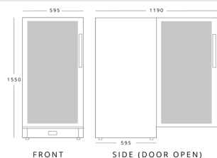
VESTFROST FZ295W H 1550mm W 595mm D 595mm
